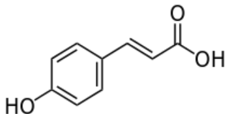
Εικόνα 5. Α) Το π-κουμαρικό οξύ είναι ένα υδροξυκινναμικό οξύ, μια οργανική ένωση που είναι ένα υδροξύ παράγωγο του κινναμικού οξέος, Β) Το χλωρογενικό οξύ (CGA) είναι ο εστέρας του καφεϊκού οξέος και του (-) - κινικού οξέος, που λειτουργεί ως ενδιάμεσο στη βιοσύνθεση λιγνίνης.
