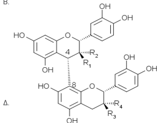
Εικόνα 4. Α) Η κερκετίνη, Β) Η τυροσόλη είναι ένα φαινυλαιθανοειδές, παράγωγο της φαινυλαιθικής αλκοόλης, φυσικό φαινολικό αντιοξειδωτικό που υπάρχει σε μια ποικιλία φυσικών πηγών, όπως π.χ. το ελαιόλαδο, Γ) Το γαλλικό οξύ (επίσης γνωστό ως 3,4,5-τριυδροξυβενζοϊκό οξύ) είναι ένα τριυδροξυβενζοϊκό οξύ, ένας τύπος φαινολικού οξέος, που βρίσκεται σε καρύδια, σουμάκ, φουντουκιά, φύλλα τσαγιού, φλοιό βελανιδιάς και άλλα φυτά, Δ) Οι προκυανιδίνες είναι μέλη της κατηγορίας φλαβονοειδών προανθοκυανιδίνης (ή συμπυκνωμένων ταννινών).
