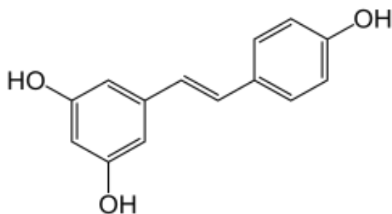
Εικόνα 7. Ρεσβερατρόλη (3,5,4'-τριϋδροξυ-trans-στιλβένιο) είναι ένα στιλβενιοειδές, ένας τύπος φυσικής φαινόλης και μια φυτοαλεξίνη (φυτό+αλεξίνη=αποκρούω, διώχνω), ουσία προστατευτική που παράγεται από πολλά φυτά ως απόκριση σε τραυματισμό ή όταν το φυτό δέχεται επίθεση από παθογόνα.
